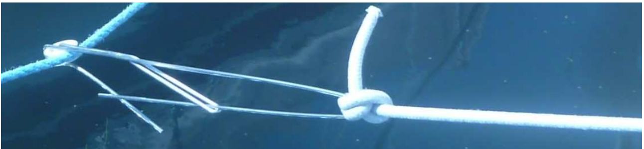
Fang-Fix-Haken Öffnen durch Ausklinken aus der doppelseitigen Führungsgabel
